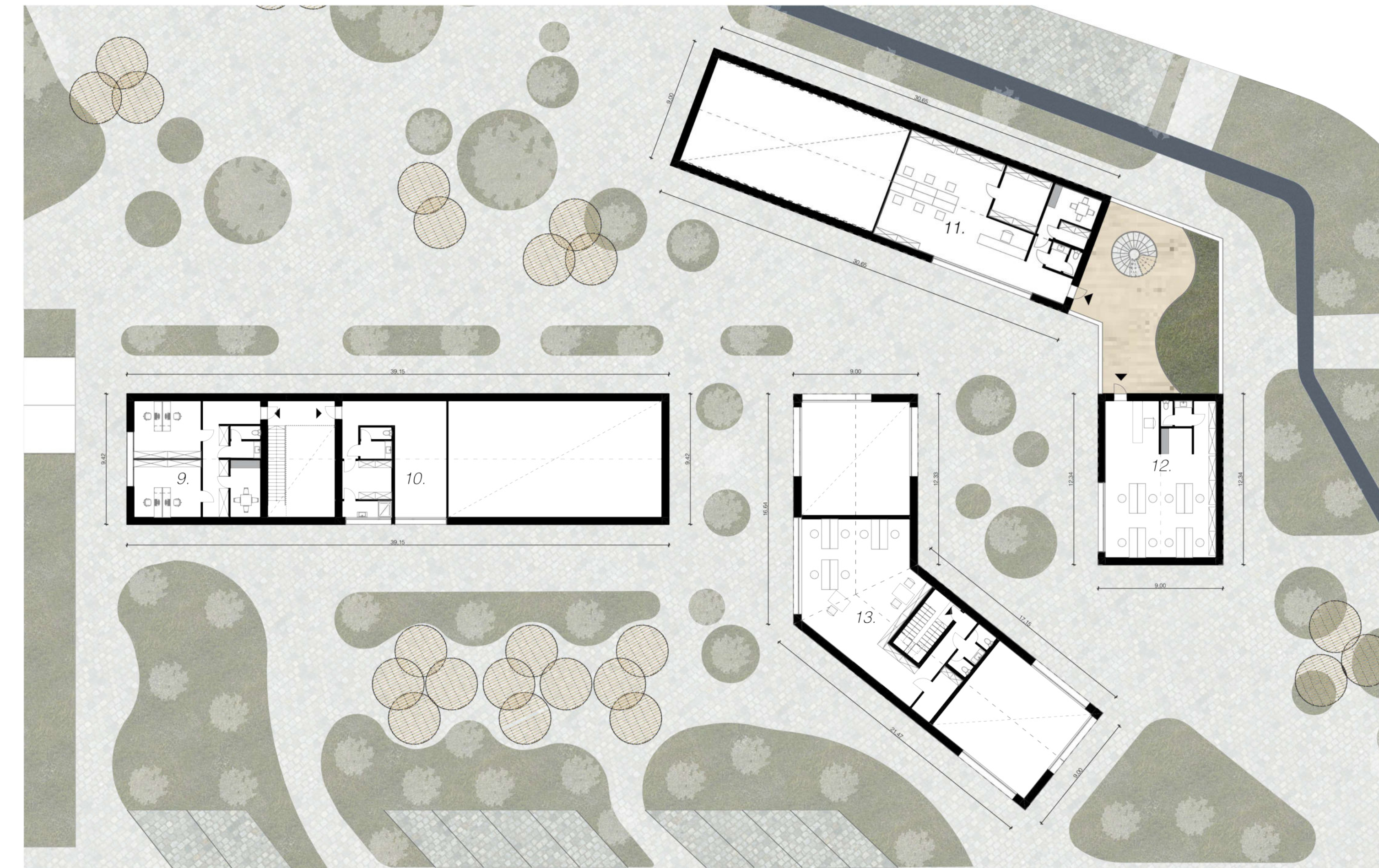
Emeleti alaprajz M 1:200
