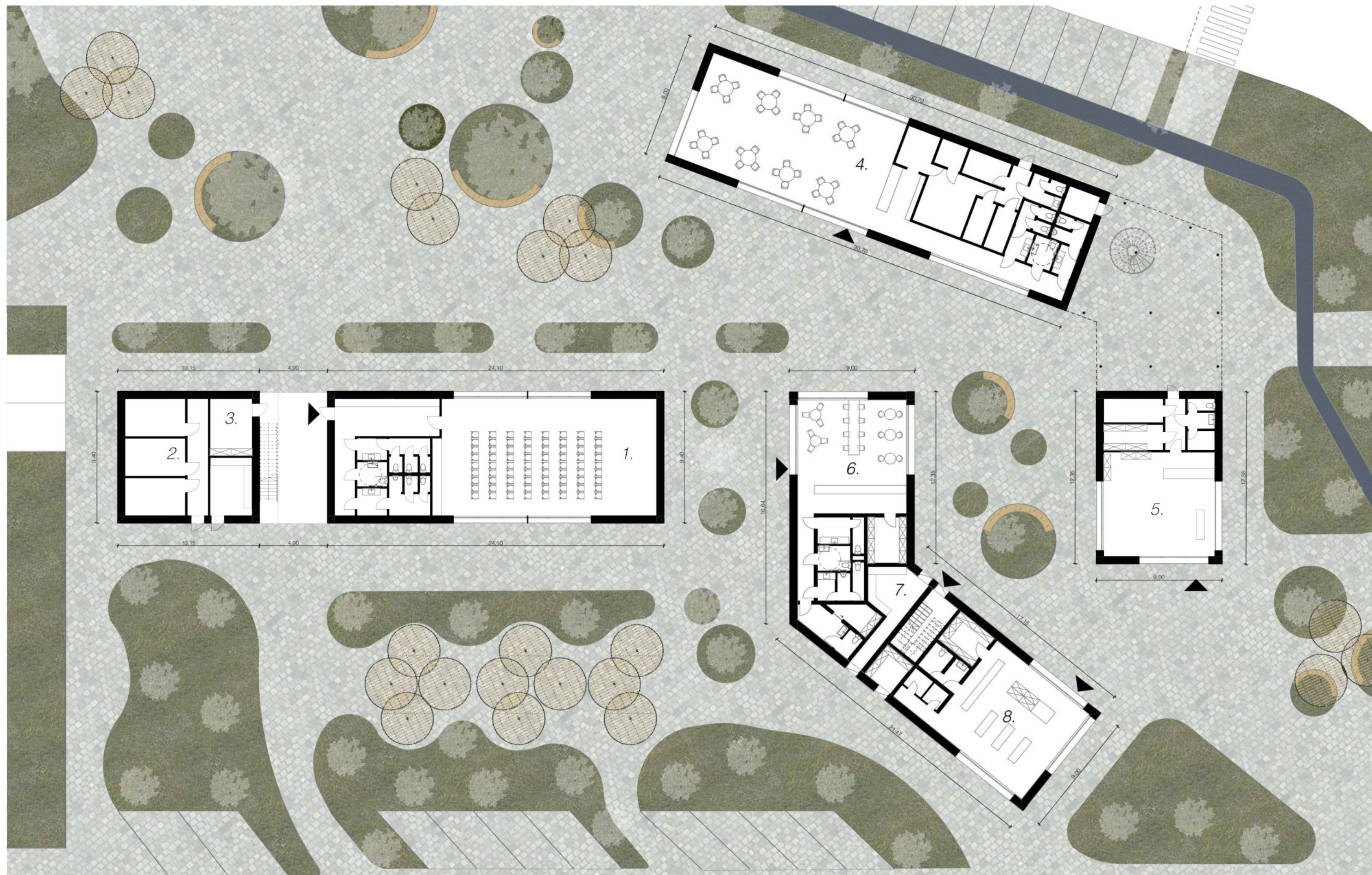
Földszinti alaprajz M 1:200
